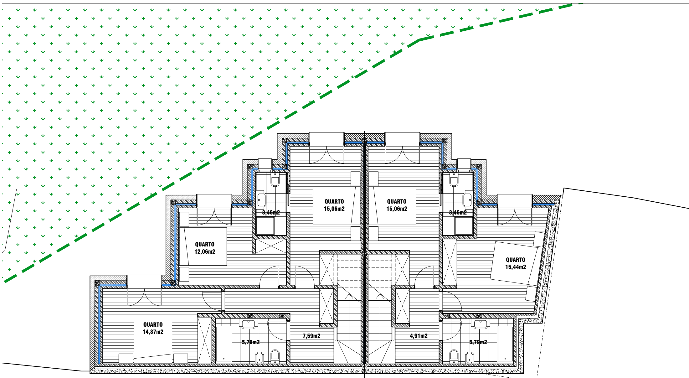
Planta da cave
