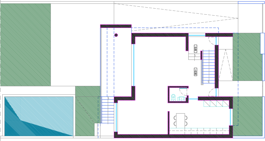
Planta do piso 0
